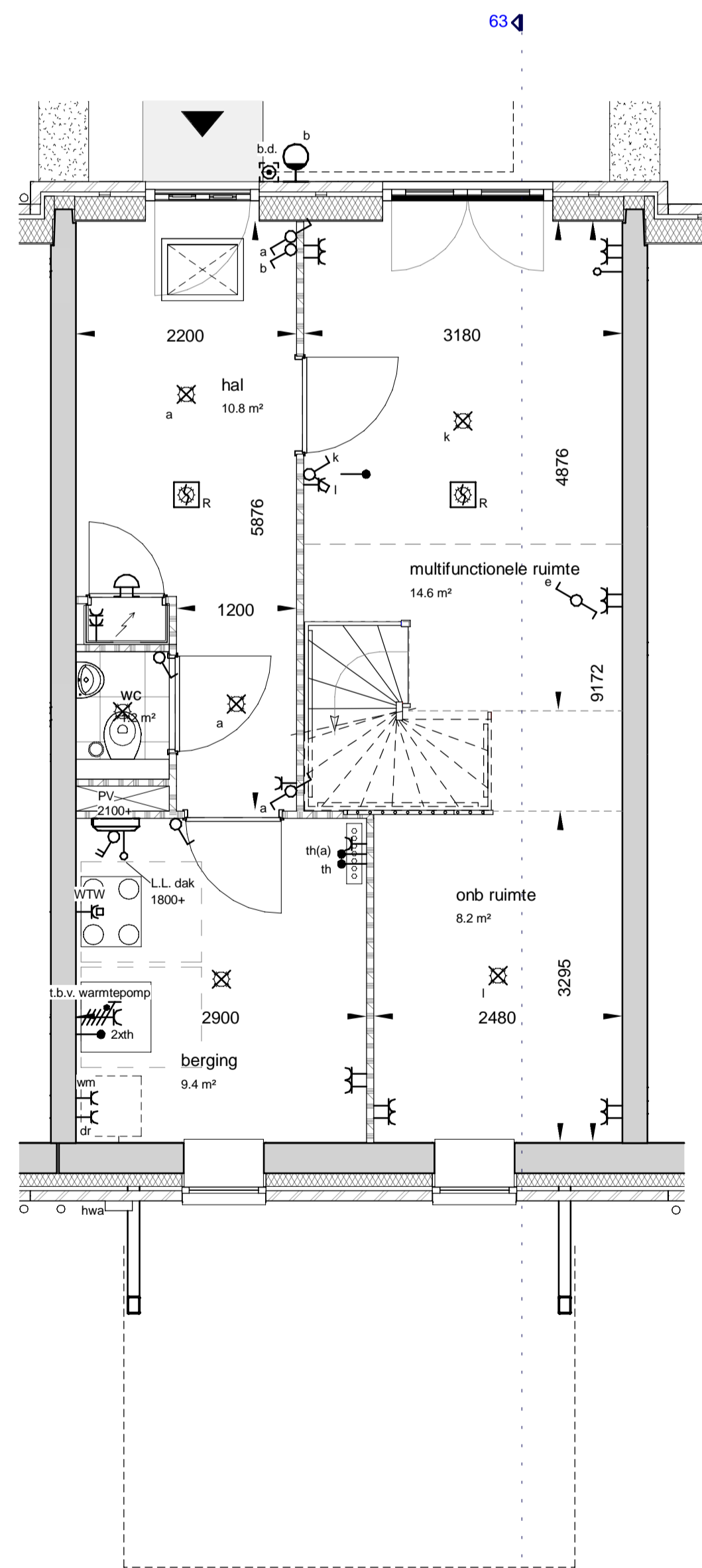
begane grond
