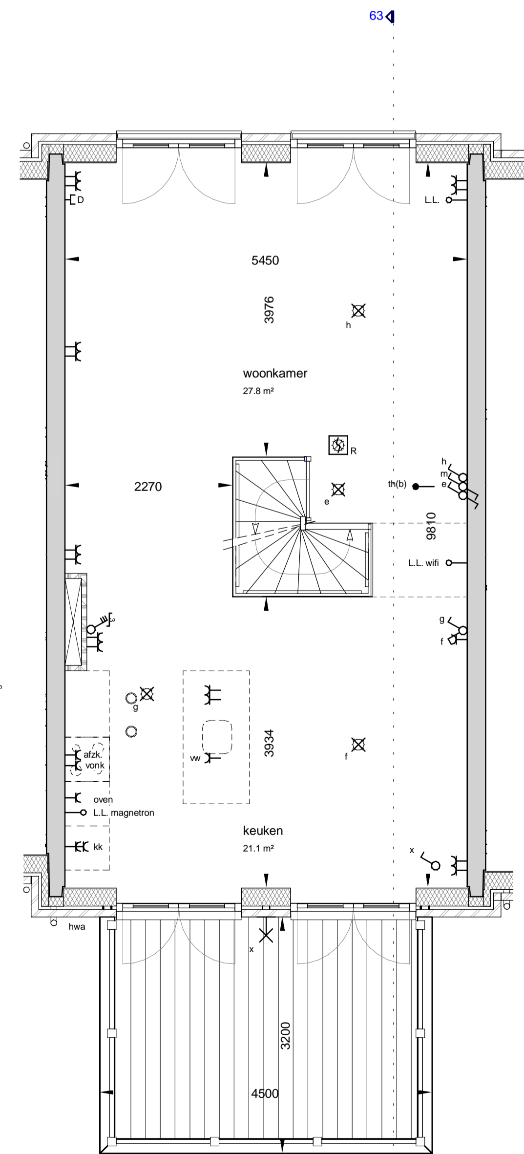
eerste verdieping
