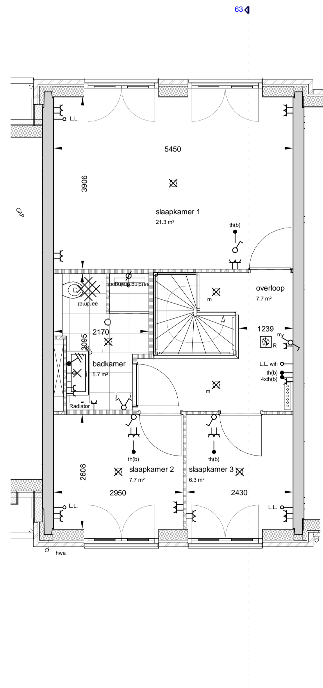
tweede verdieping
