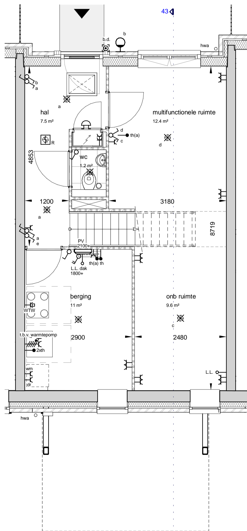
begane grond
