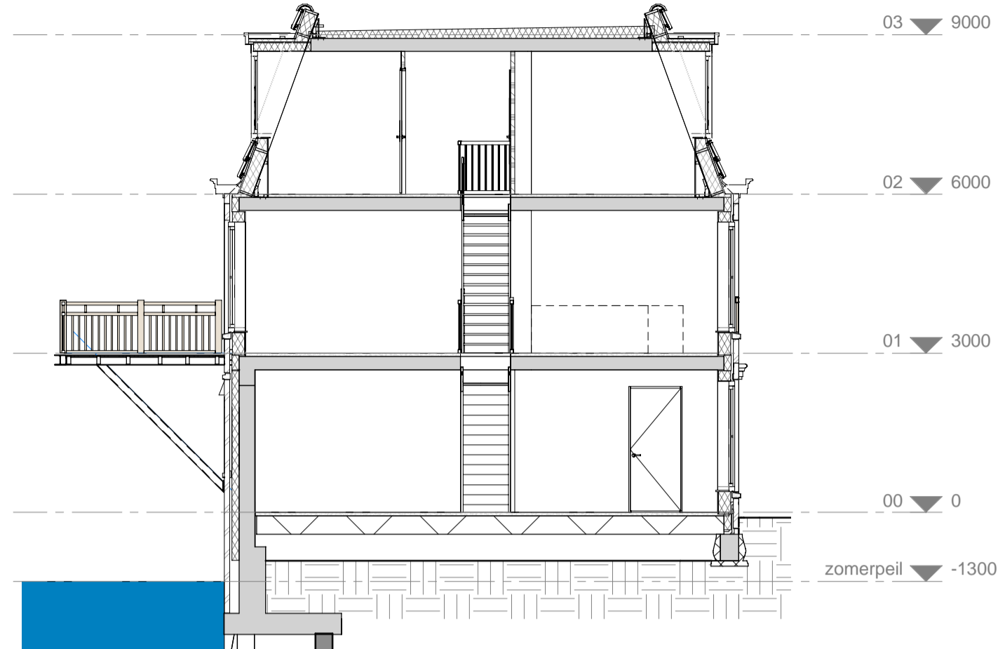
doorsnede
