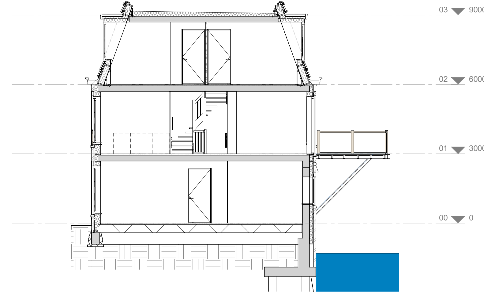
doorsnede
