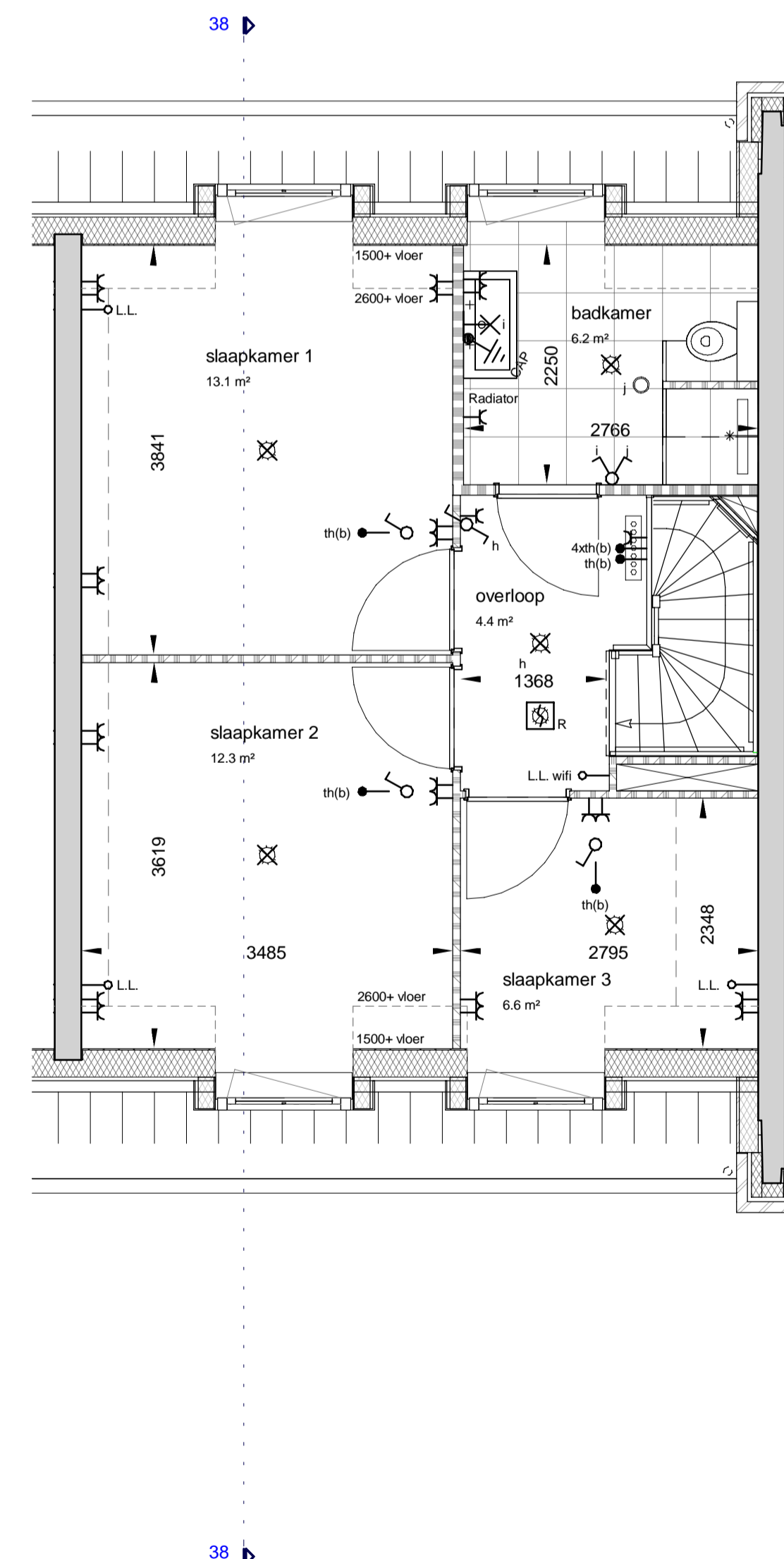
tweede verdieping
