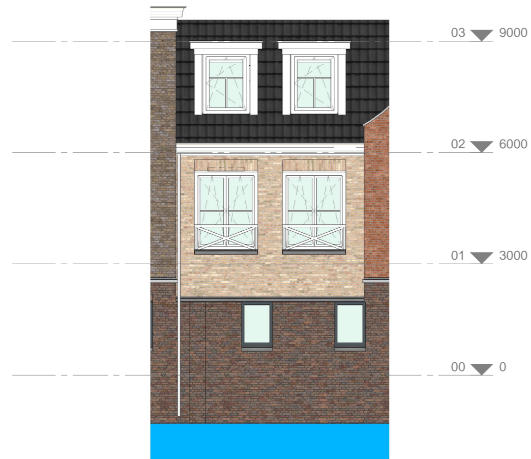
watergevel
