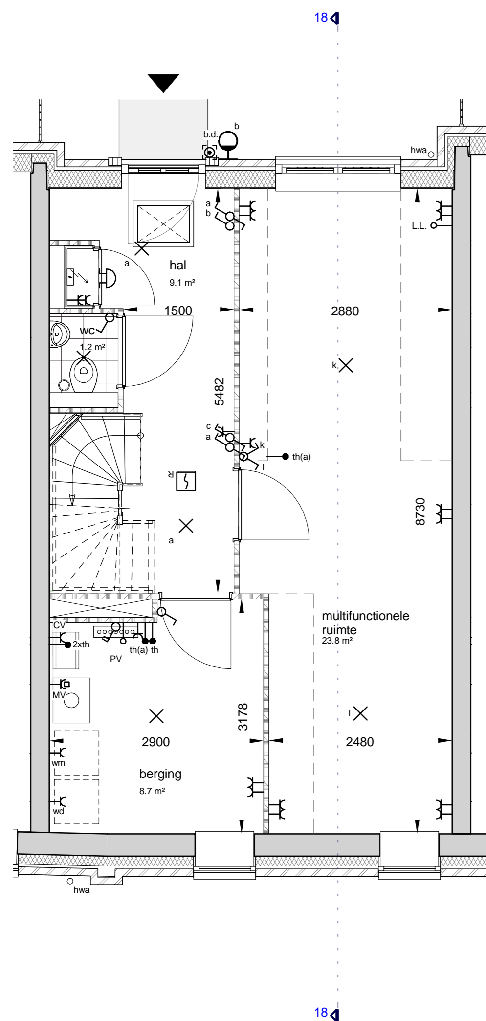
begane grond
