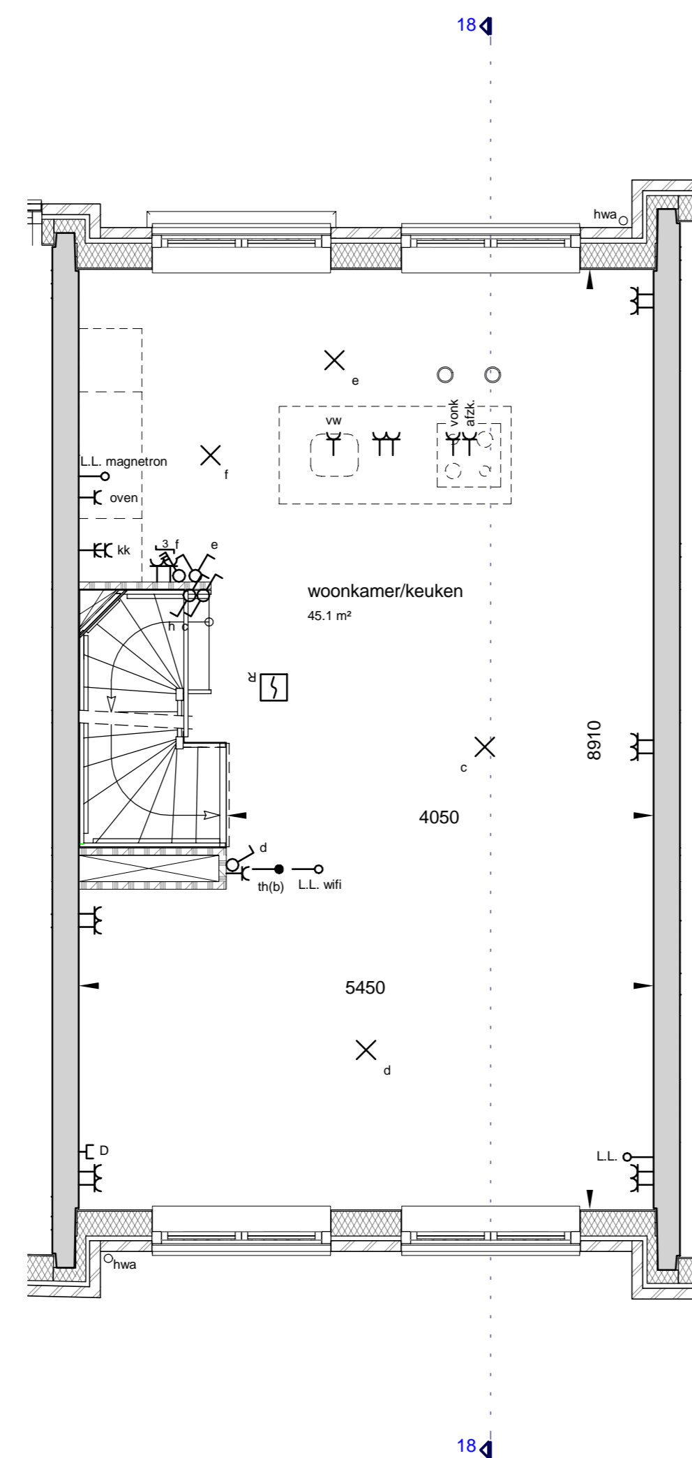
eerste verdieping
