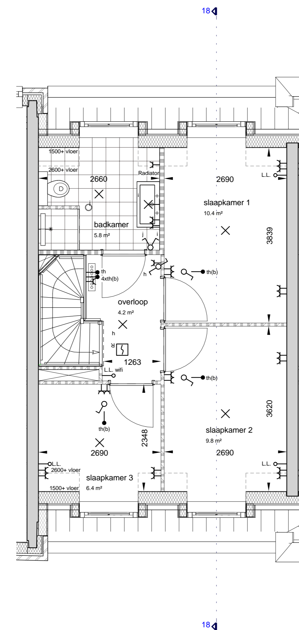
tweede verdieping
