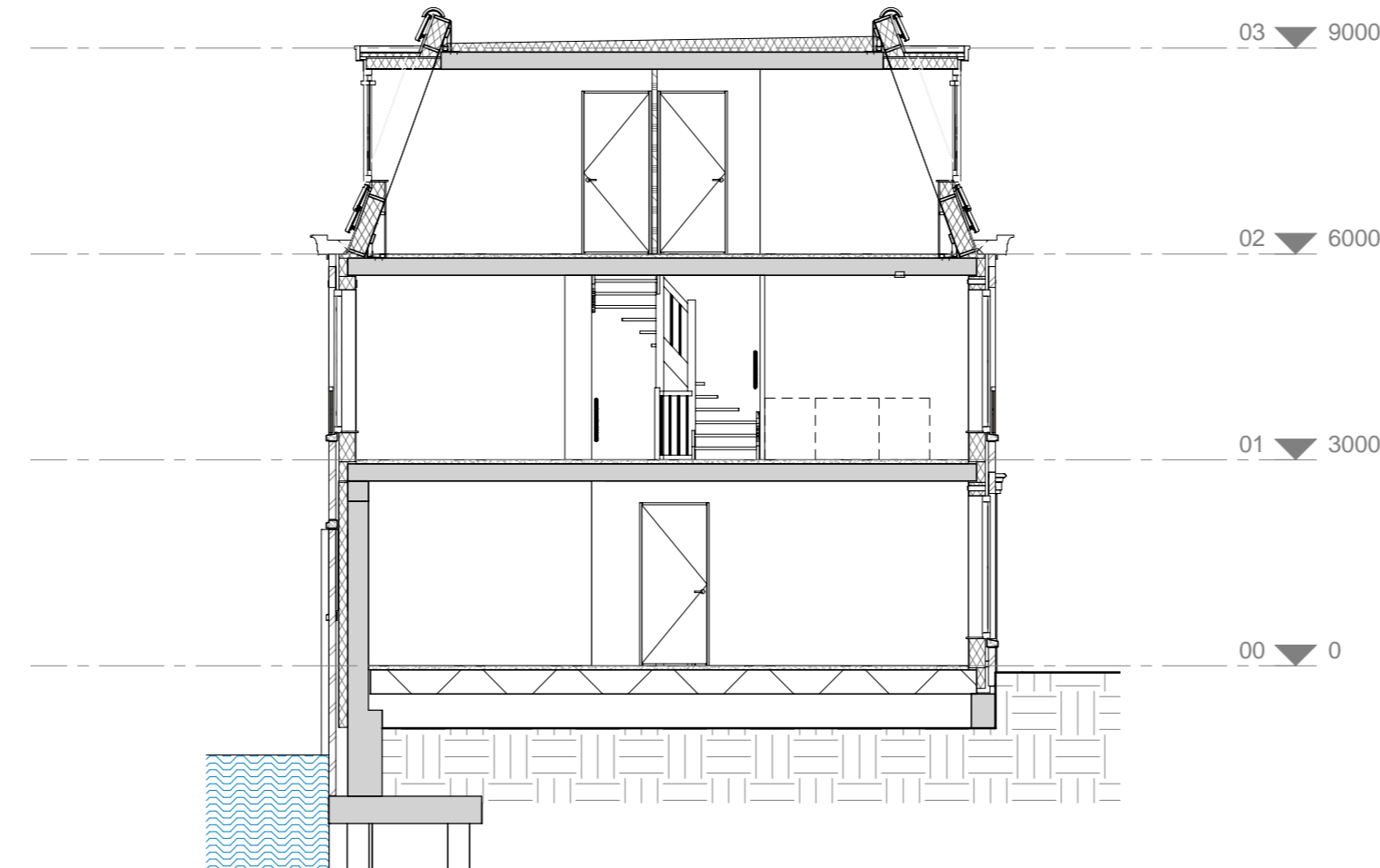
doorsnede
