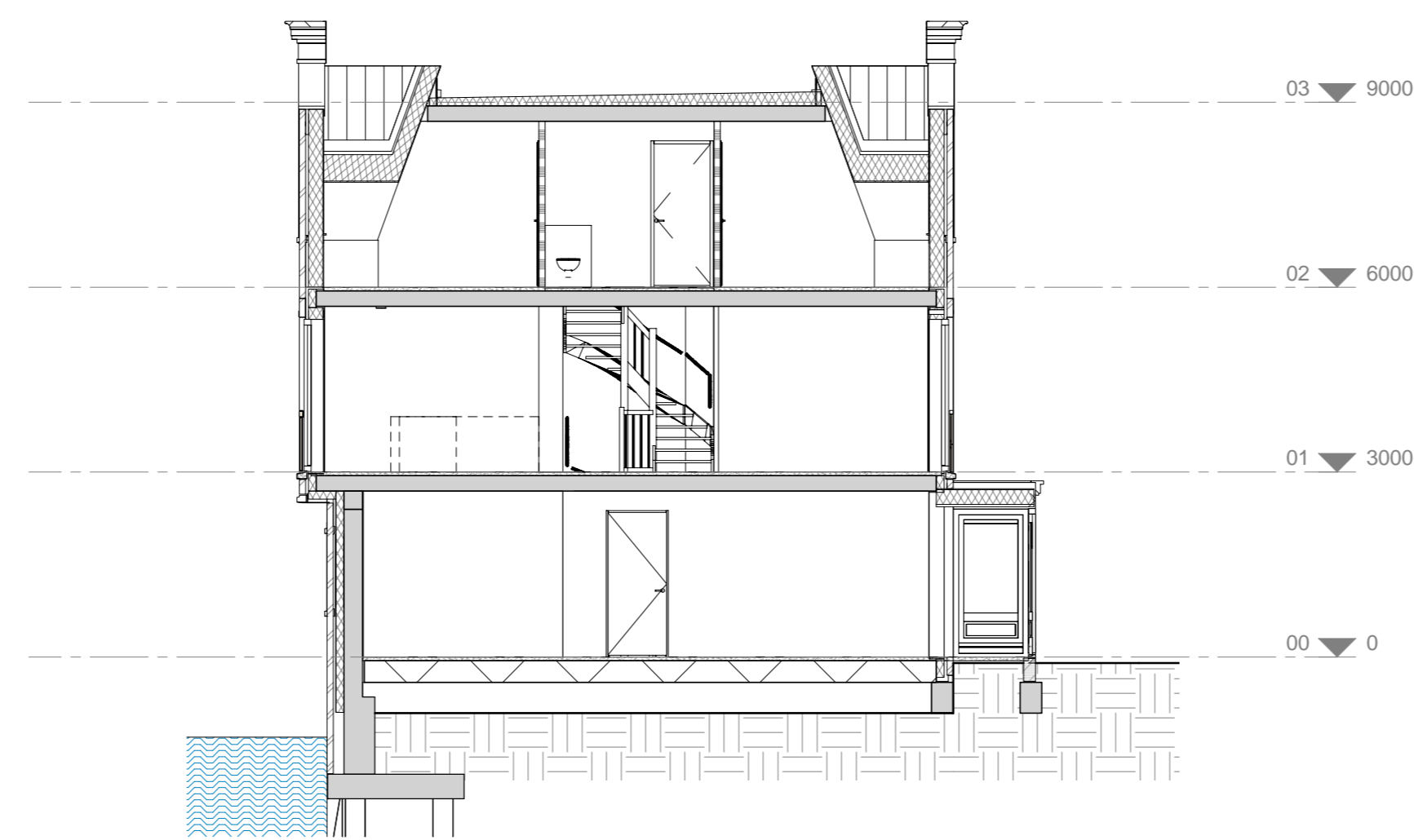
doorsnede
