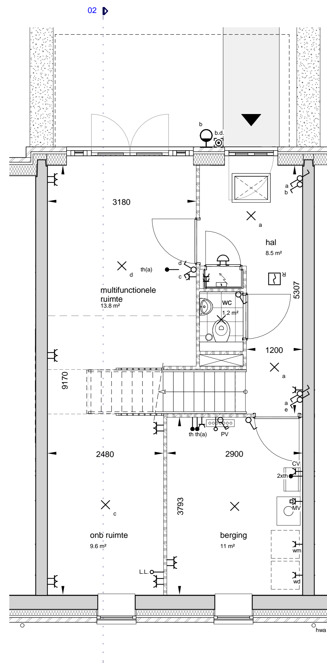
begane grond
