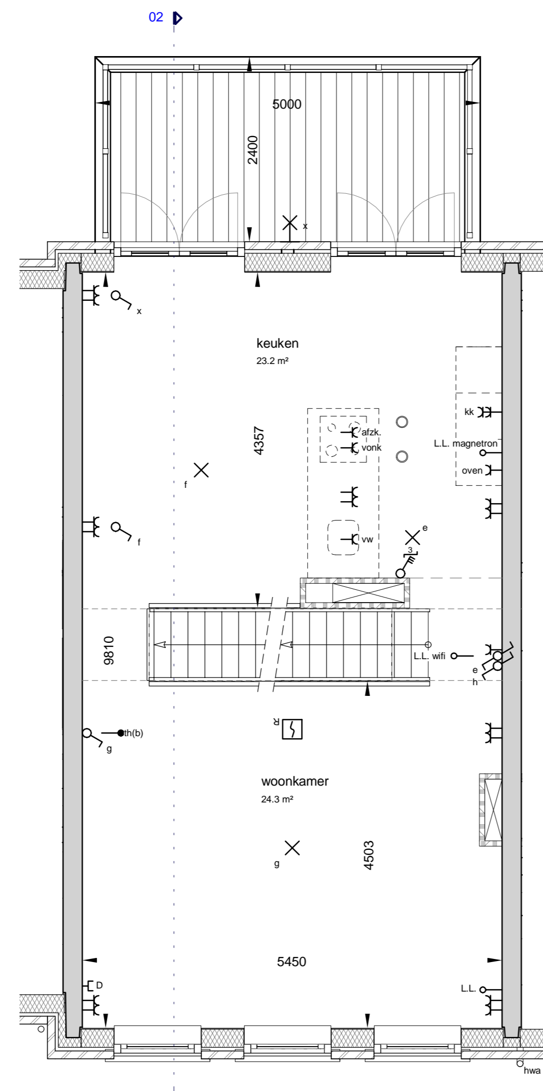
eerste verdieping
